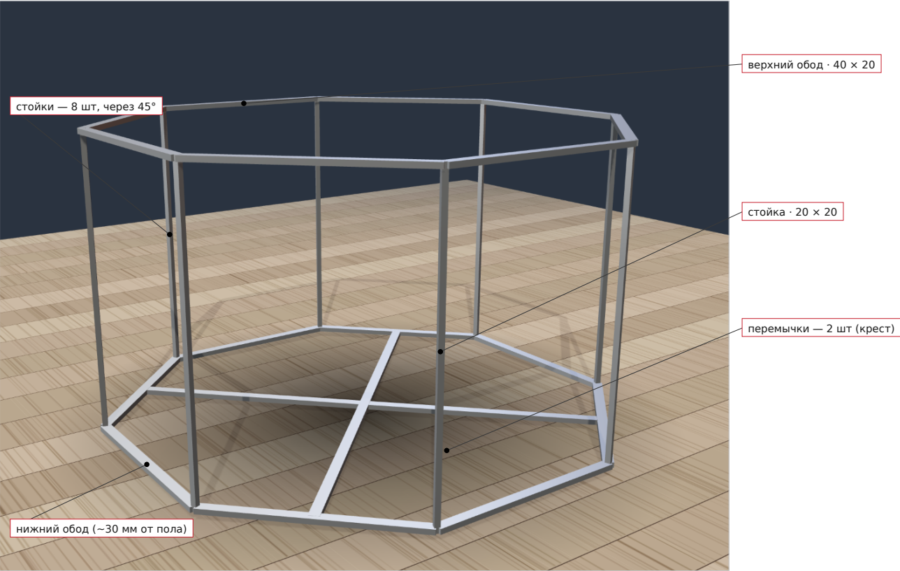
КАРКАС · перспектива 3/4
